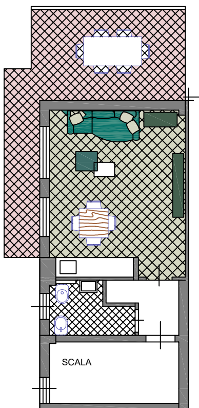
PIANO PRIMO
